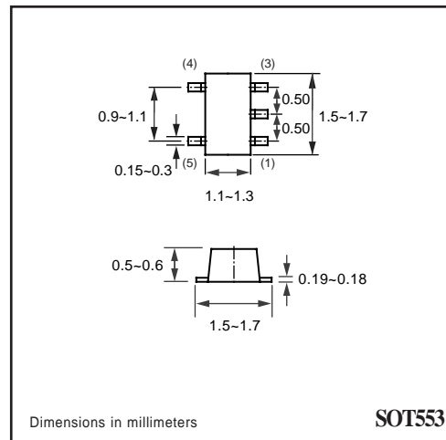
SOT553
